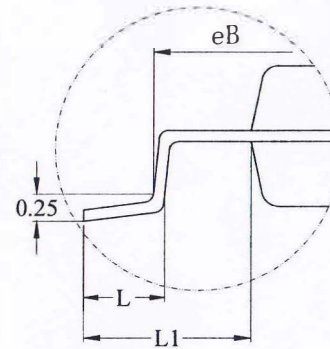
DETAIL: F
